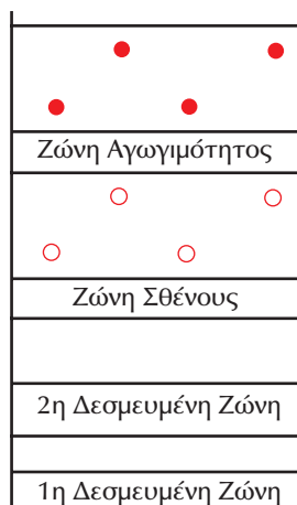
Σχήμα 2.1.3 Διάγραμμα ενεργειακών ζωνών ενός υλικού
